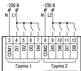
Рисунок 6 – Подключение дискретных датчиков с питанием 230 В
