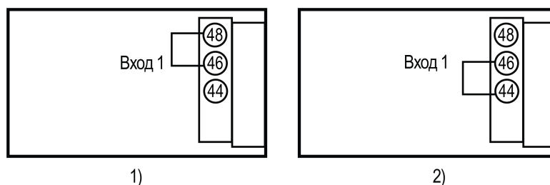
Рисунок 7.8 – Установка перемычки
