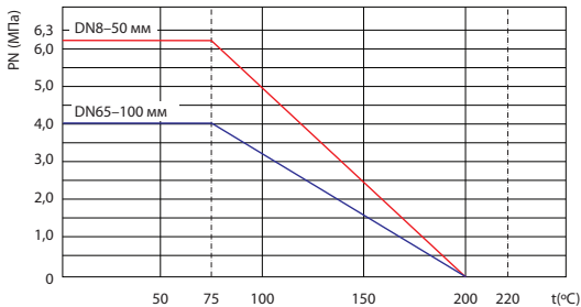
Диаграмма «Температура-Давление»
