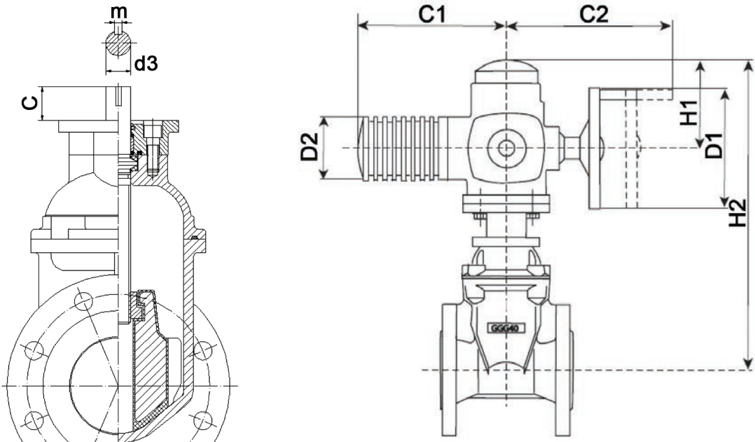
Исполнение с электроприводом
