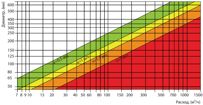
Диаграмма подбора
