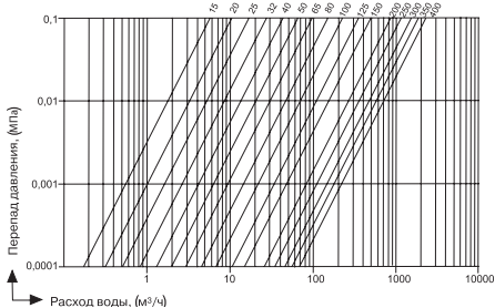
Диаграмма перепада давления для фильтра стандартного исполнения
