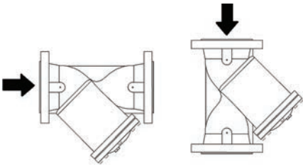
Способы установки фильтра
