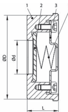
Исполнение для DN 15–100
