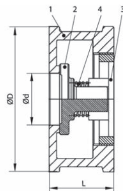
Исполнение для DN 125–300
